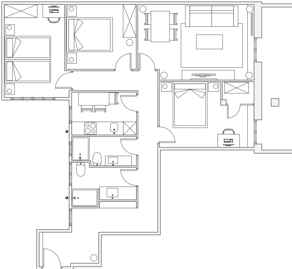
PLANTA DE DISTRIBUCION REFORMADA ESCALA 1/100
